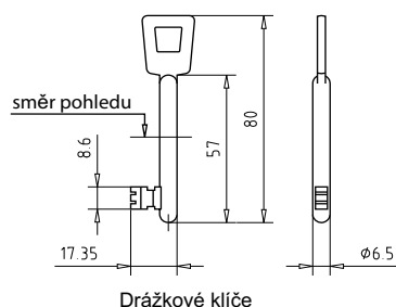
Drážkové klíče
