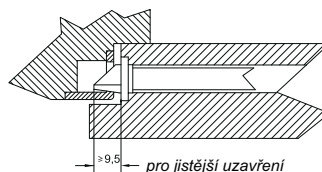
zadlabací zámek s pomocnou střelkou
