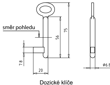
Dozické klíče
